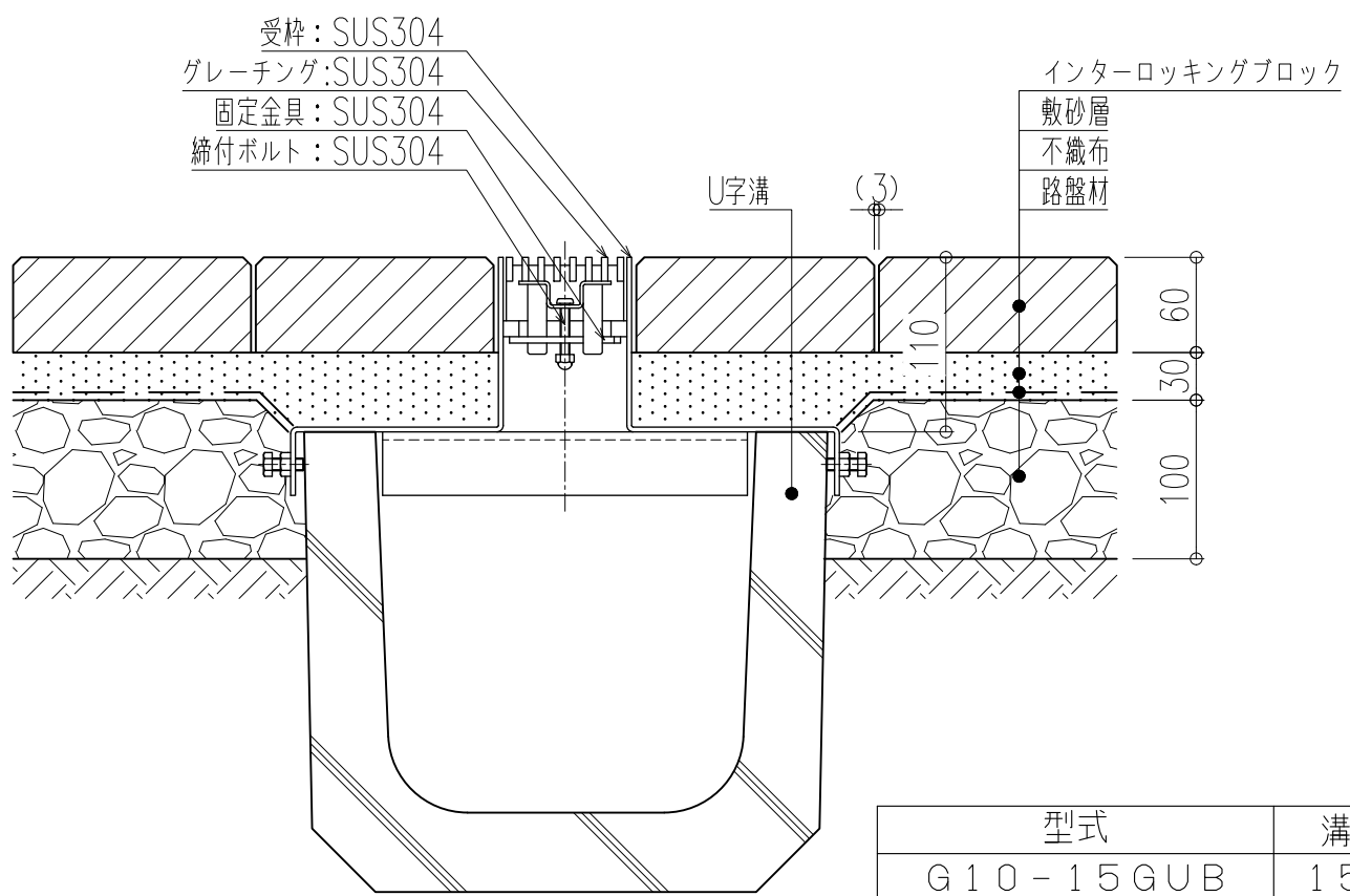
施工参考図
